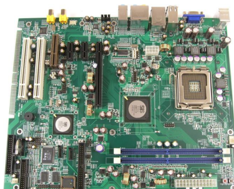
PC alaplap
